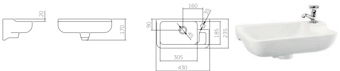
L.100 lavatório pequeno
