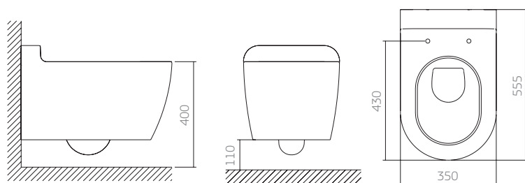
P.192 bacia convencional suspensa
