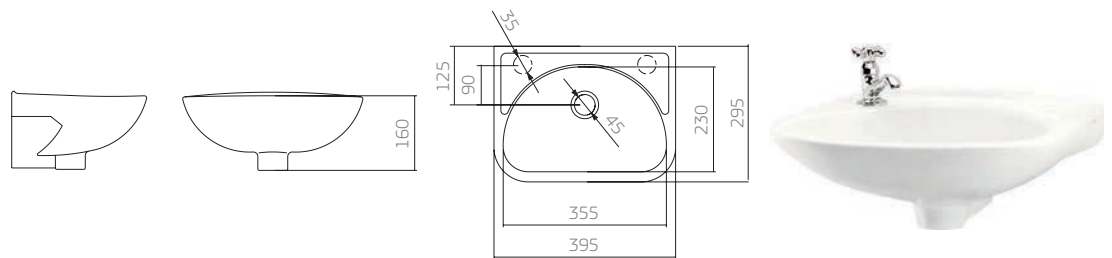
L.15 lavatório pequeno
