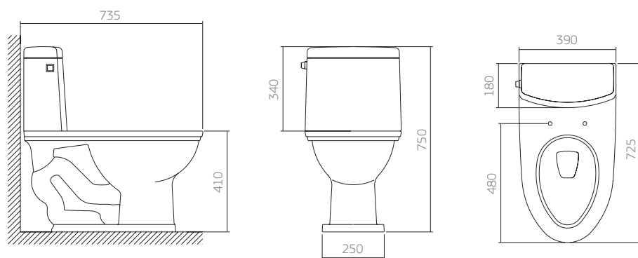
P.143 bacia monobloco e assento plástico slow close
