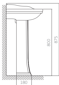
L.25 (lavatório) C.25 (coluna) lavatório com coluna
