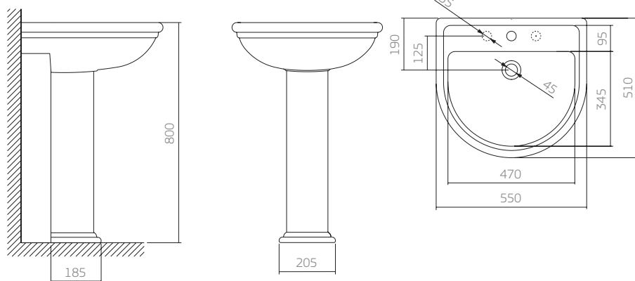
L.2 (lavatório) C.2 (coluna) lavatório com coluna
