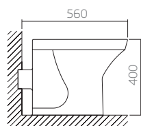
P.131 bacia convencional com saída horizontal
