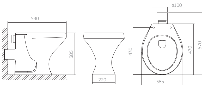
P.90 bacia convencional com saída horizontal
