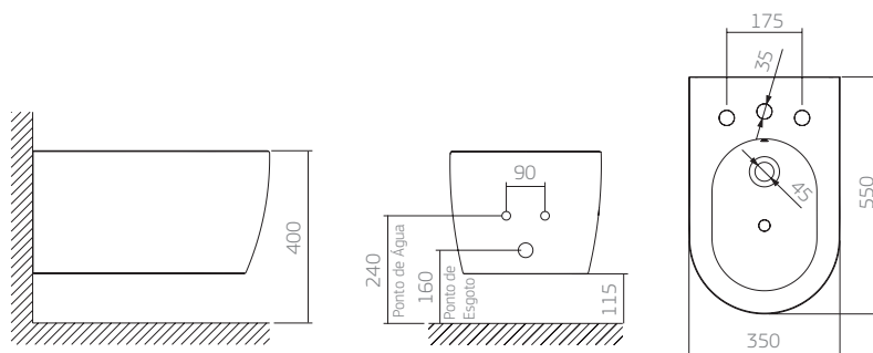
B.192 bidê suspenso (3 furos)
