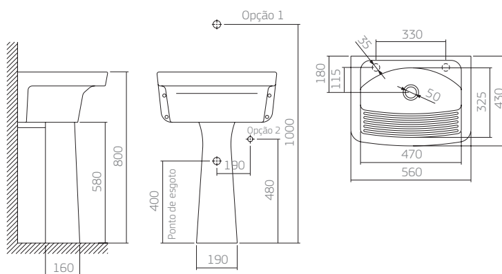
TQ.01 tanque capacidade total: 18 litros CT.11 coluna para TQ.01
