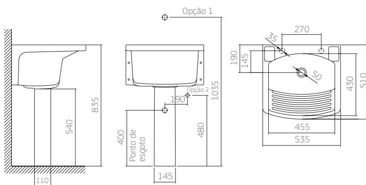
TQ.02 tanque capacidade total: 30 litros CT.25 coluna para TQ.02 e TQ.03
