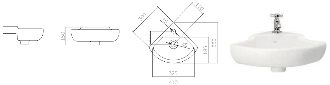
L.101 lavatório de canto
