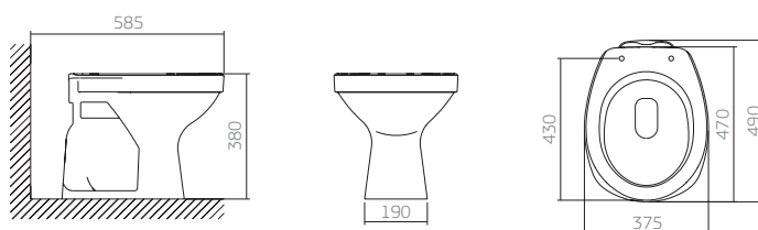
P.76 bacia convencional
